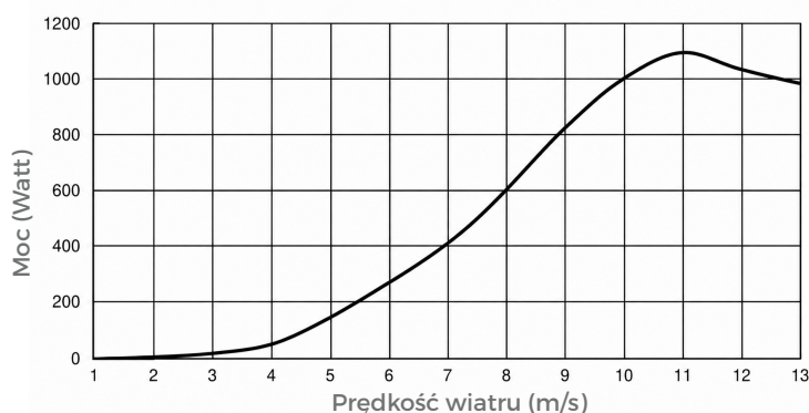
KRZYWA MOCY
