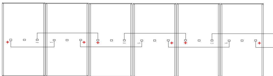
Connexion horizontale des modules
