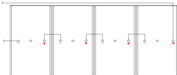
Assemblage des modules par la méthode Leapfrog (Portrait)
