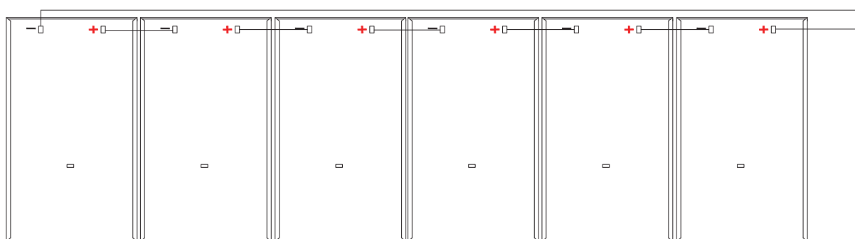
Leapfrog-Verkabelung (Hochformat)
