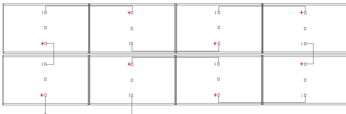
Connexion horizontale des modules
