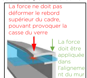
Figure 1a: Position de la Force de serrage de la bride
