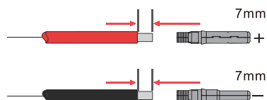
Rysunek 4.1-1 Kable PV i wtyczki PV
