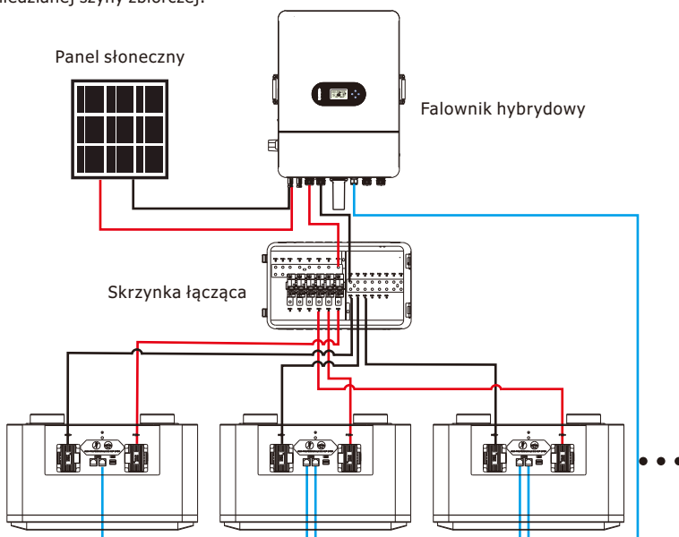
Rysunek 3-2 Schemat połączenia wielu baterii w układzie równoległym
