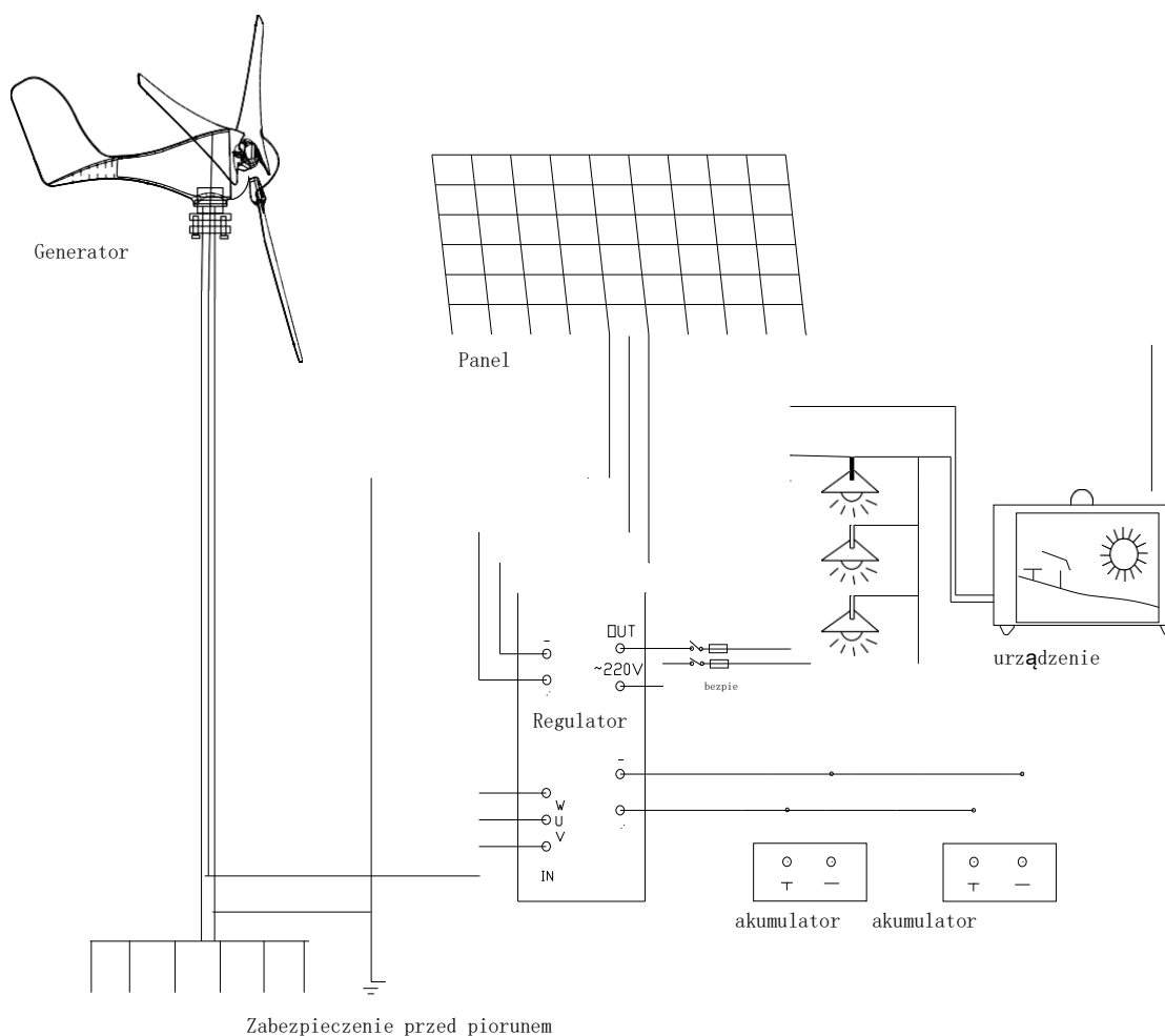
Schemat połączeń turbiny wiatrowej,
