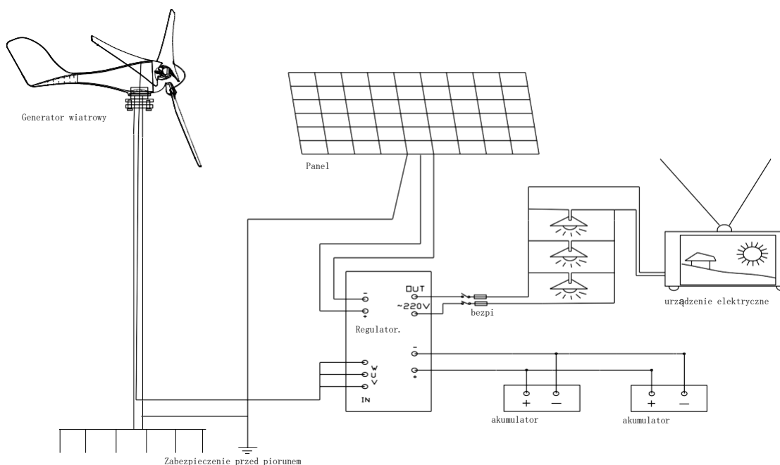
Schemat połączeń turbiny wiatrowej, panelu fotowoltaicznego i urządzenia elektrycznego
