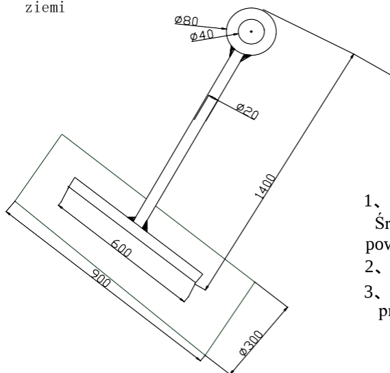
Rysunek 1: Wykonanie kopca wzmocnionej ziemi
