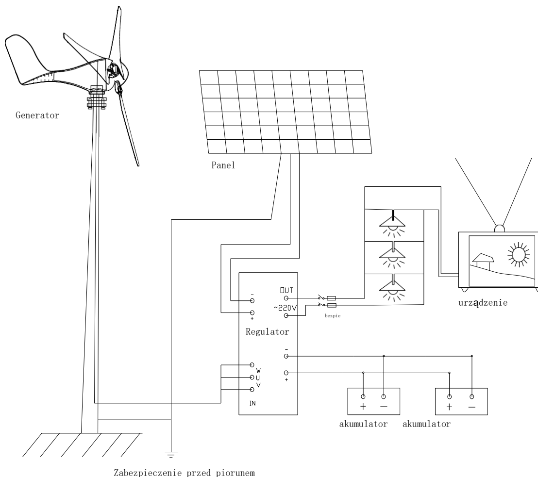
Schemat połączeń turbiny wiatrowej, panelu fotowoltaicznego i urządzenia elektrycznego
