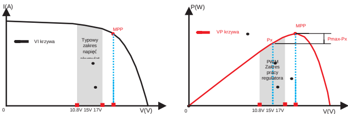
Wykres krzywej I-V nominalnej mocy wyjściowej 12 V modułu.
